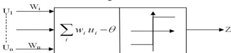
شکل ۱. نرون مصنوعی با تابع آستانه
