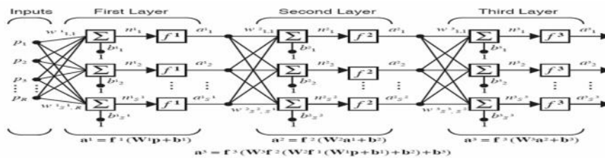
شکل ۳- پرسپترون چند لایه
